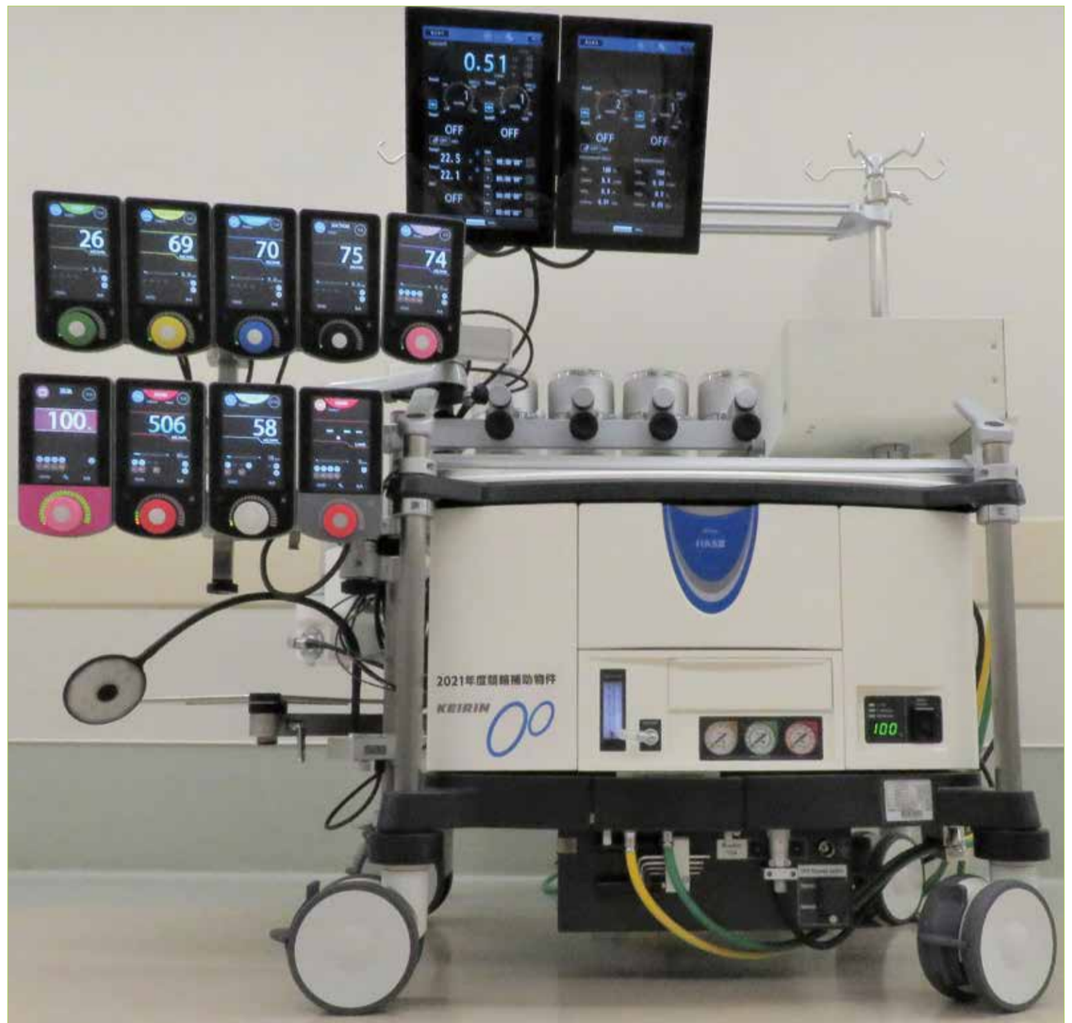
メラ人工心肺装置HASⅢ
